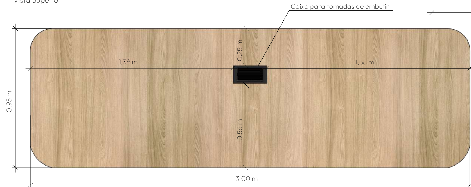
Vista Superior
